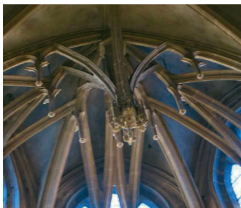
Vûtes de la cathédrale. La clé-pendante surplombe l'abside.
